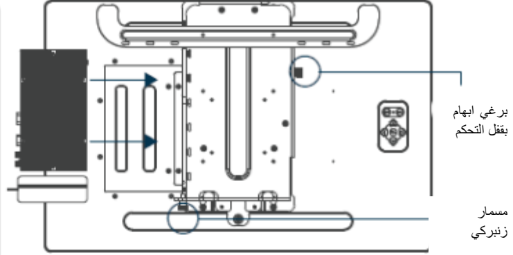
2 حرك وحدة التحكم في الحامل عن طريق محاذاة المسارات الموجودة على الحامل بمسامير الكتف الموجودة في الجزء السفلي من وحدة التحكم. اربط الكابلات بوحدة التحكم المضمنة مع الشاشة. قم بتأمين وحدة التحكم باستخدام مسمار الإيهام.
